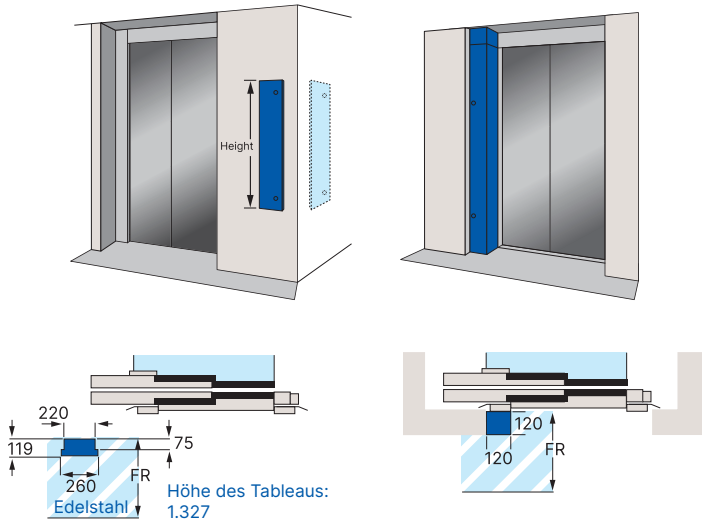
Wandmontiertes Wartungstableau
